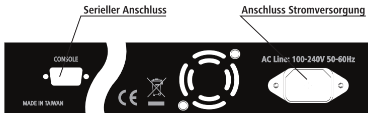
LANCOM GS-2352 Rückseite
