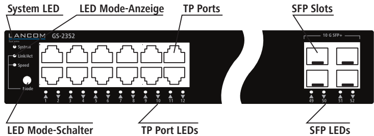
LANCOM GS-2352 Vorderseite
