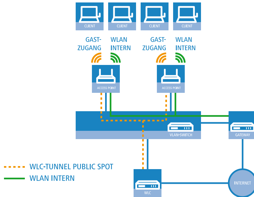
Abbildung 12: "Anwendungsbeispiel WLAN-Controller mit Public Spot"
