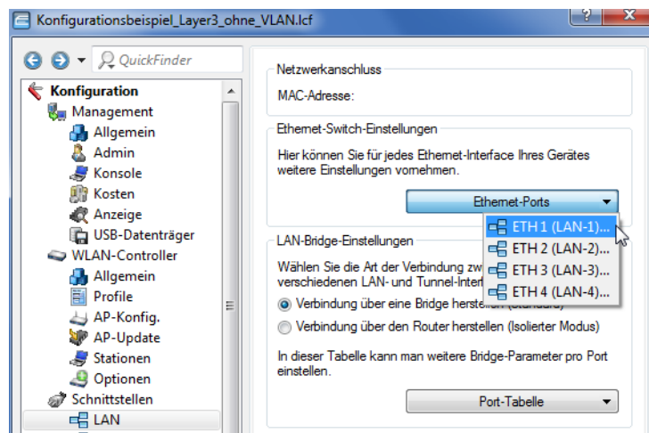
Abbildung 8: "Ethernet-Einstellungen für Overlay-Netze"
