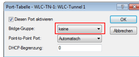
Abbildung 19: "Port-Einstellungen für Public-Spot-APs"
