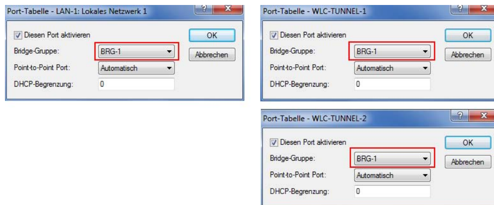
Abbildung 9: "Port-Einstellungen für Overlay-Netze"
