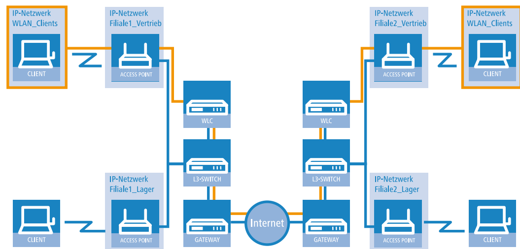
Abbildung 2: "Overlay-Netzwerk über mehrere IP-Netzwerke hinweg"
