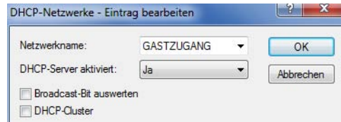
Abbildung 10: "DHCP-Netzwerk für Overlay-Netze"
