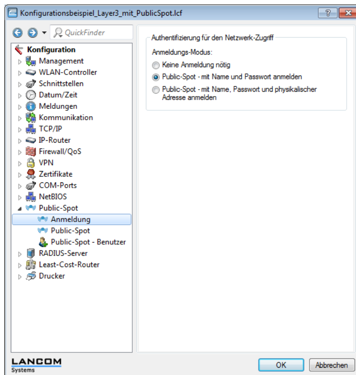
Abbildung 26: "Aktivierung der Anmeldung über den Public-Spot"
