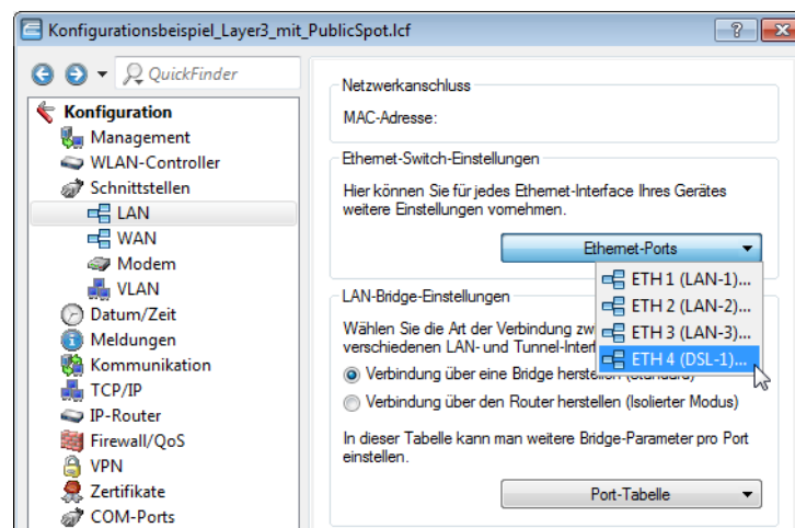
Abbildung 18: "Ethernet-Einstellungen für Public-Spot-APs"
