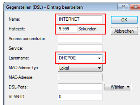
Abbildung 20: "Gegenstelle für Internet-Zugang"
