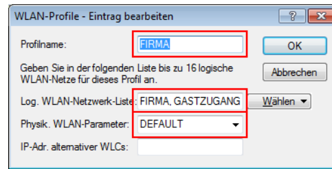
Abbildung 16: "WLAN-Profil für Public-Spot-APs"
