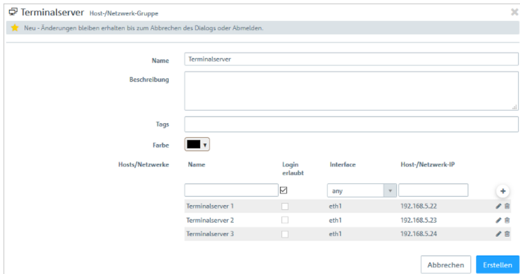
Abbildung 35: Objekteinstellungen – Terminalserver
