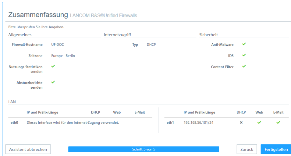
Abbildung 9: Zusammenfassung der gemachten Einstellungen
