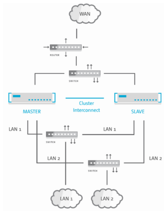
Abbildung 18: Beispiel-Netzwerk für Hochverfügbarkeit
