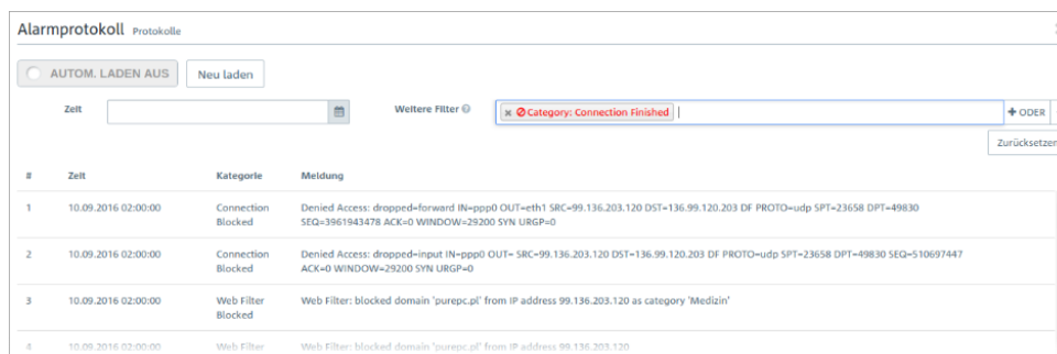
Abbildung 22: Alarmprotokoll mit angewandtem Filter
