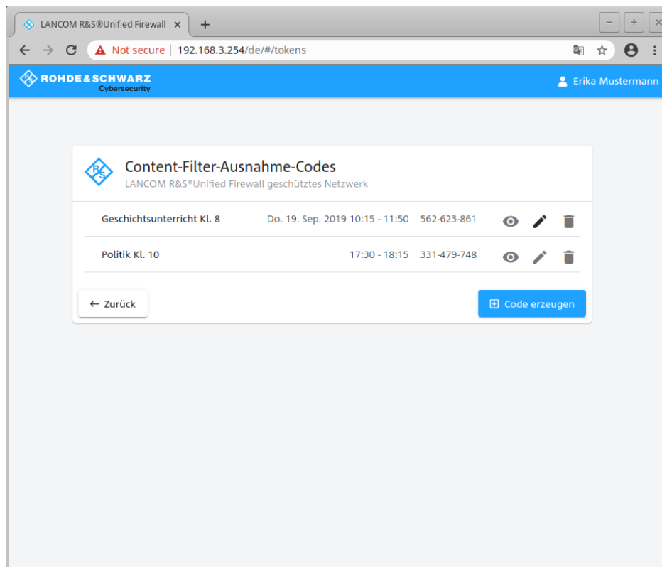
Abbildung 25: Ausnahme-Code: Managementmodus
