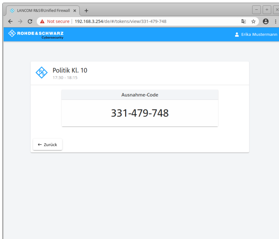
Abbildung 24: Ausnahme-Code: Präsentationsmodus
