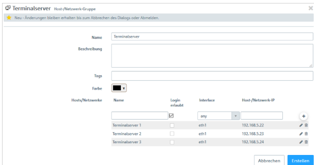
Abbildung 37: Objekteinstellungen – Terminalserver
